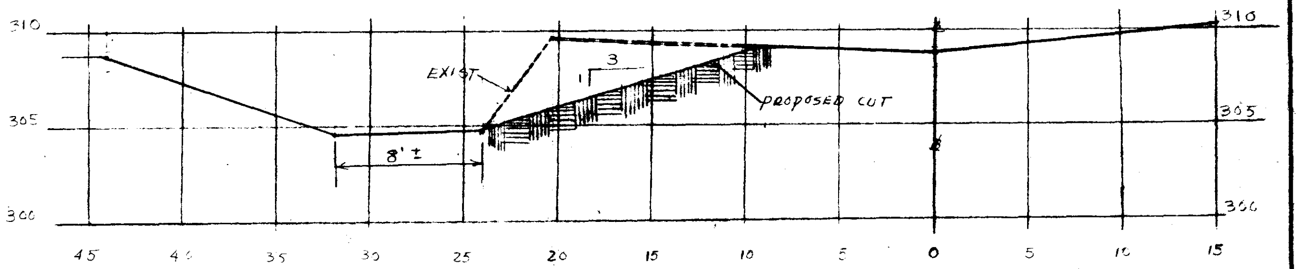
STA. NO. 7+00 1" = 5' HORIZ 1" = 5' VERT
