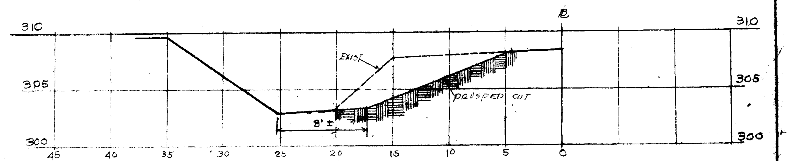
STA. NO. 7+59+00 1" = 5' HORIZ 1" = 5' VERT
